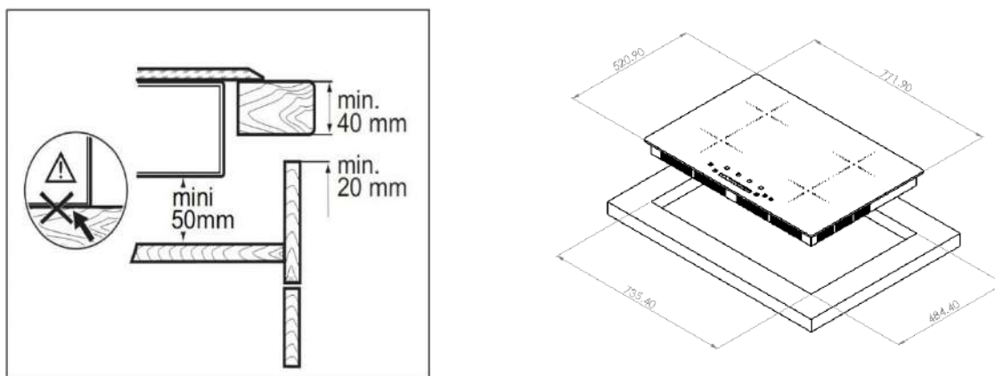
FIGURA 4 (DIMENSIONES MODELO INDUZIONE 76).
